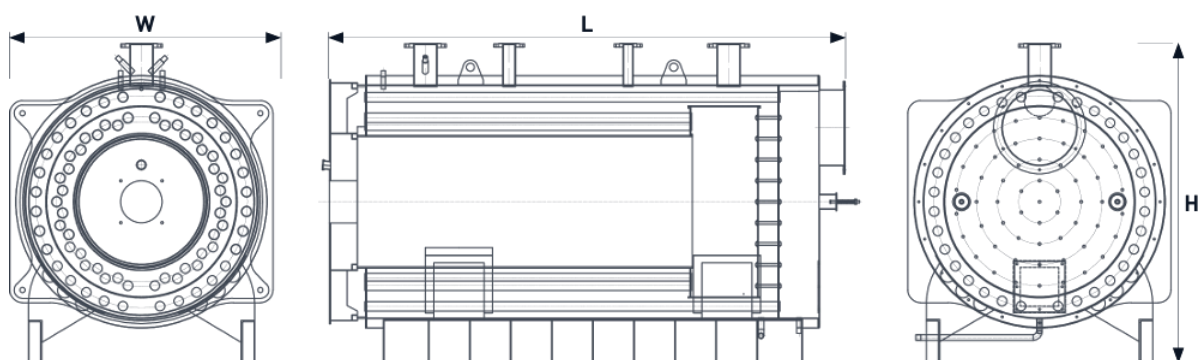
ГАБАРИТНЫЙ ЧЕРТЁЖ
